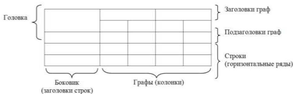
Рисунок 1 – Построение таблиц
